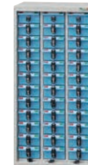
DF-MP-36C(36 格) 45W×24.5D×96.5H cm
